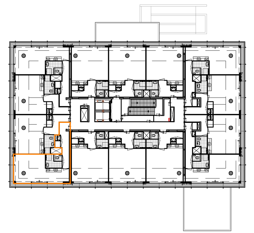
Overzichtsplattegrond 1e verdieping schaal 1:350
